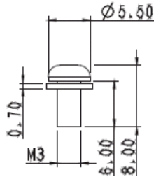
브라켓 A 잠금 나사
