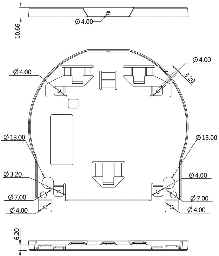
브라켓 A - 장치면
