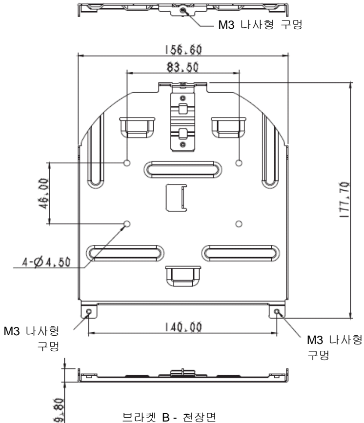
브라켓 B - 천장면
